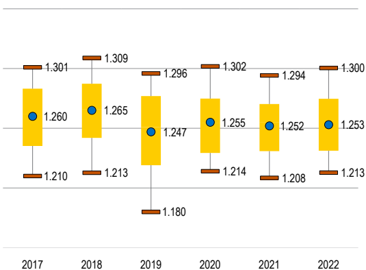
Densidad verdadera (g/cm 3 )
